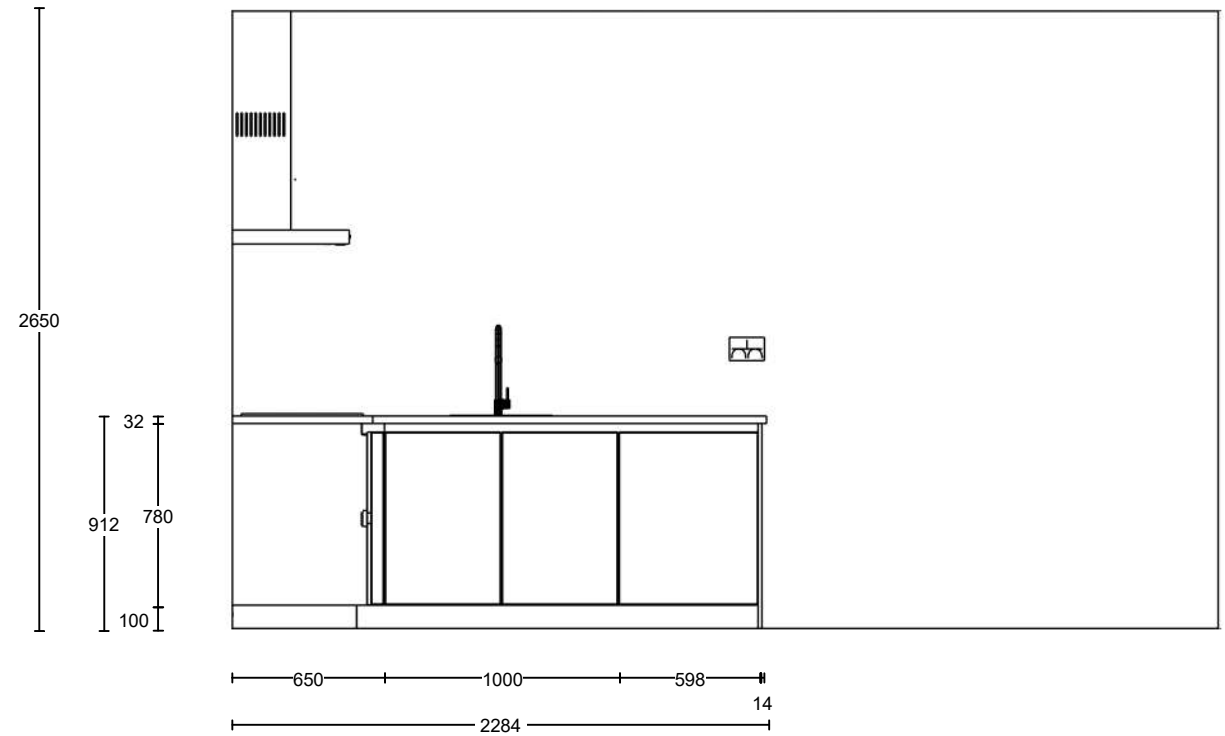
Vooraanzicht wand 2
